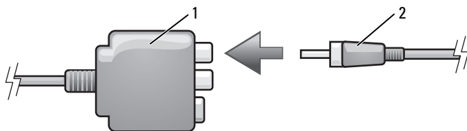
1 复合视频适配器 2 S/PDIF 数字音频电缆
