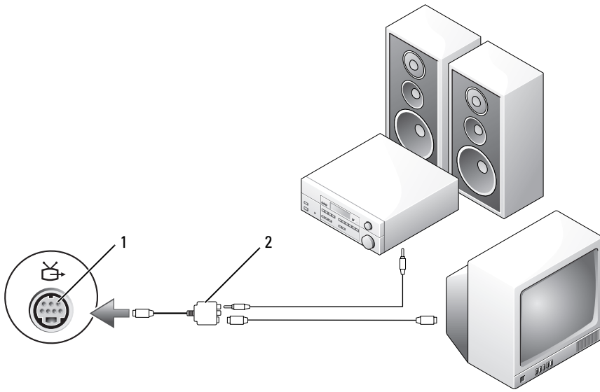
1 S 视频电视输出连接器 2 复合视频适配器
